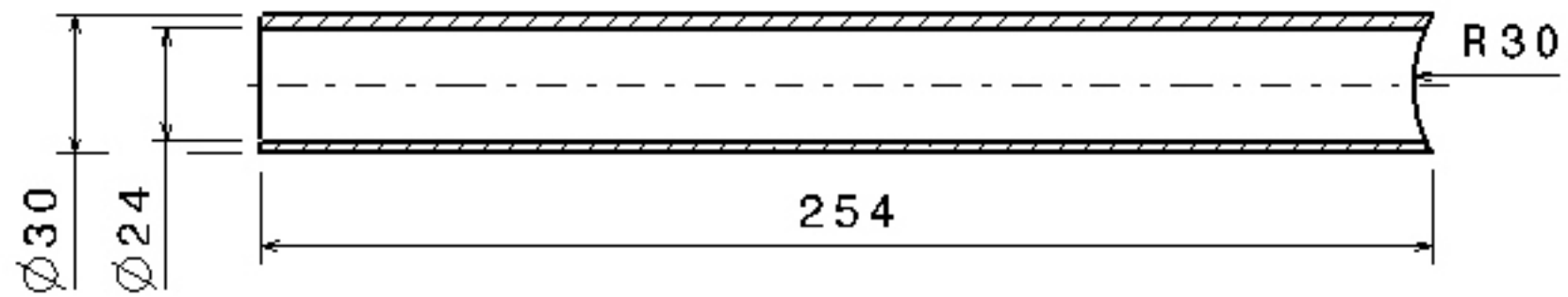
doorsnede A-A
